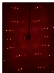
单晶衍射图
