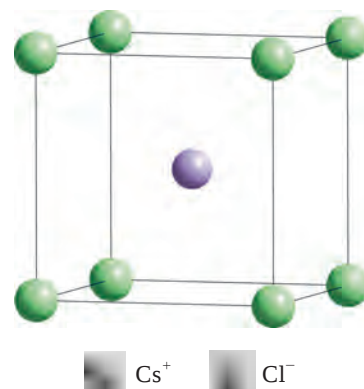
图 3.12 CsCl 晶体的晶胞
