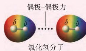
图 2.20 取向力
