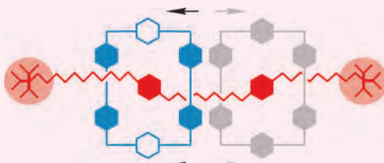
(b) 轮烷
