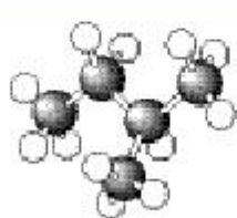
异戊烷
